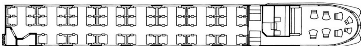
ETR.250 - Carrozza 4 Scala 1:160
